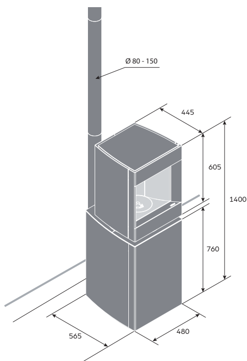
Stûv P-10 con base de acero
