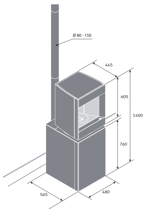
Stûv P-10 con base para revestir
